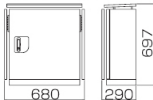
■電源BOX外観図 (停電対応オプション)
